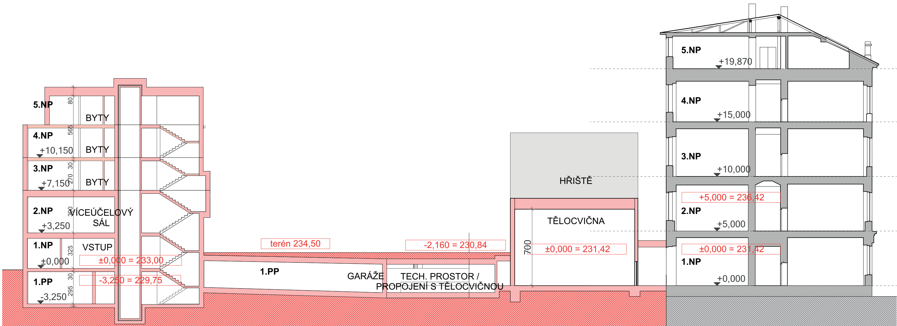
ŘEZ CELKOVÝ-MAXIMÁLNÍ ZÁSTAVBA 1:200
