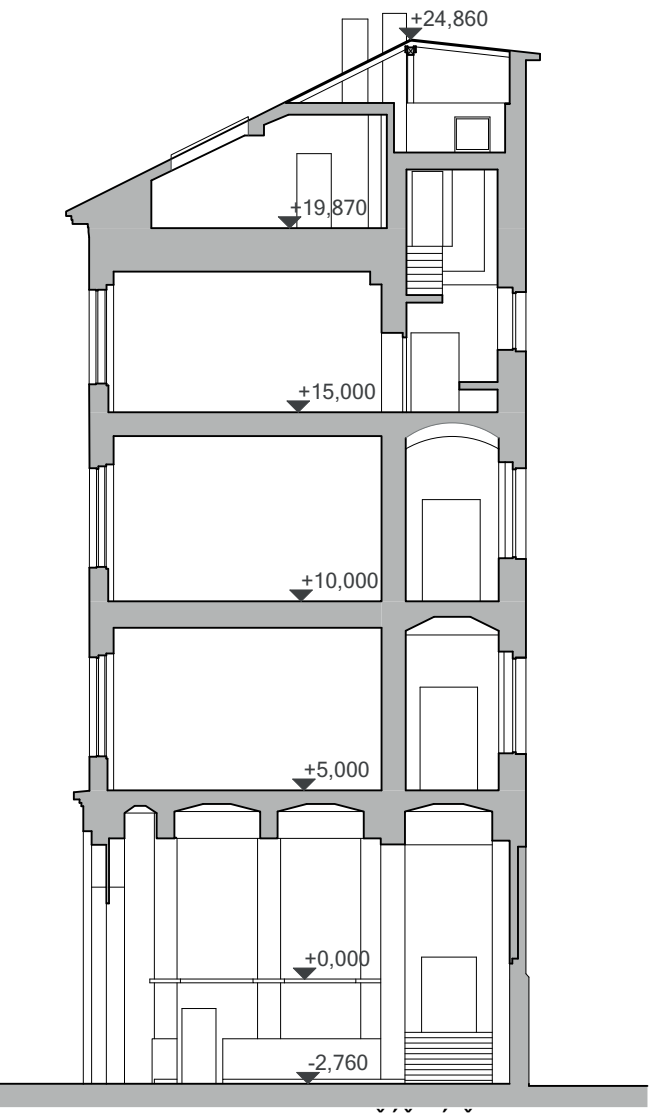
PŘÍČNÝ ŘEZ B-B'
