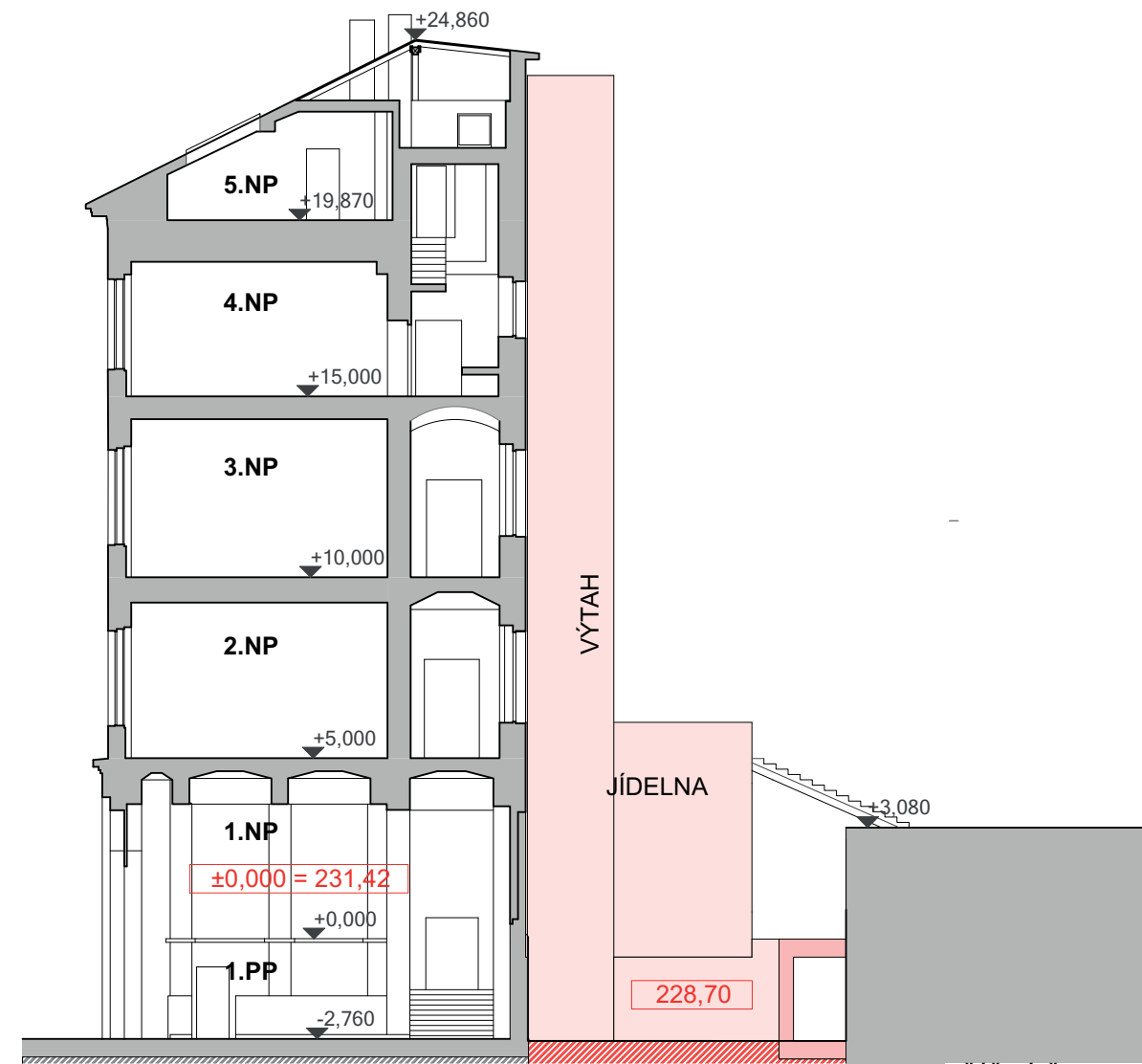
PŘÍČNÝ ŘEZ B-B
