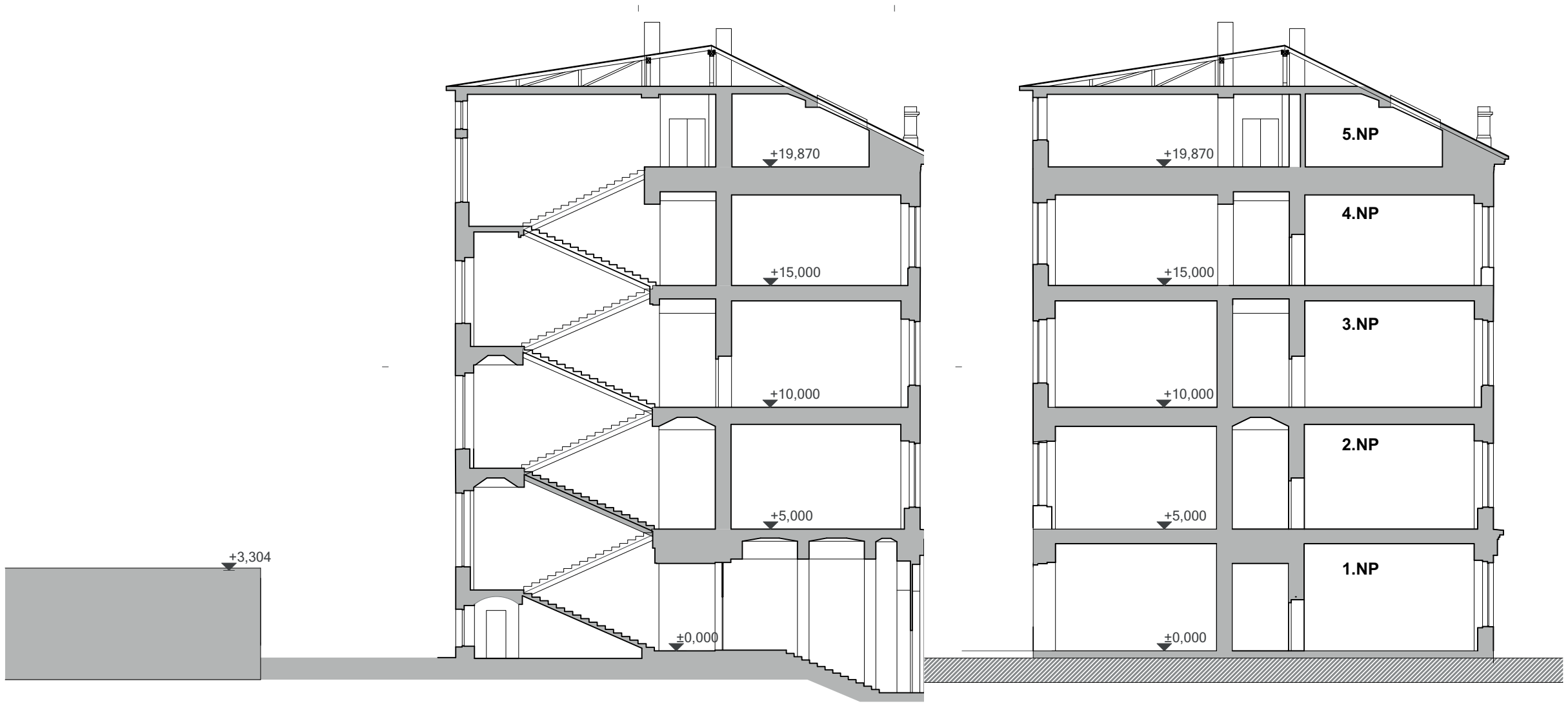
PŘÍČNÝ ŘEZ A-A'
