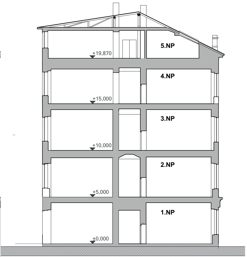
PŘÍČNÝ ŘEZ A-A'
