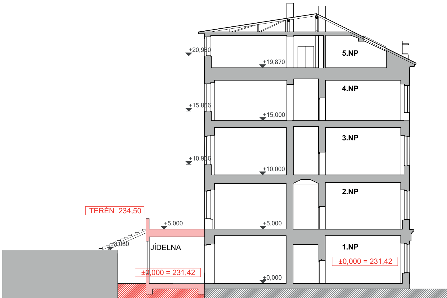
PŘÍČNÝ ŘEZ DOSTAVBOU JÍDELNY
